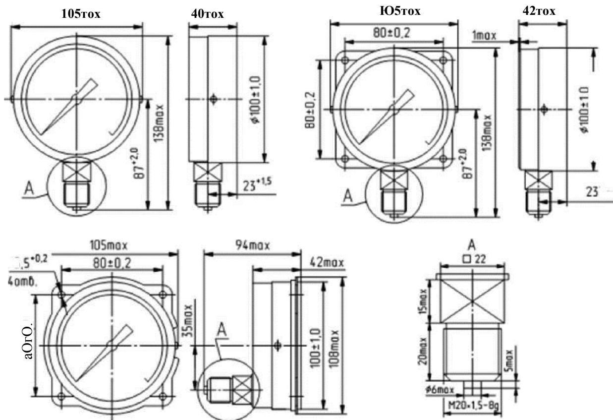
Габаритные и присоединительные размеры МПЗА-У2-Кс
